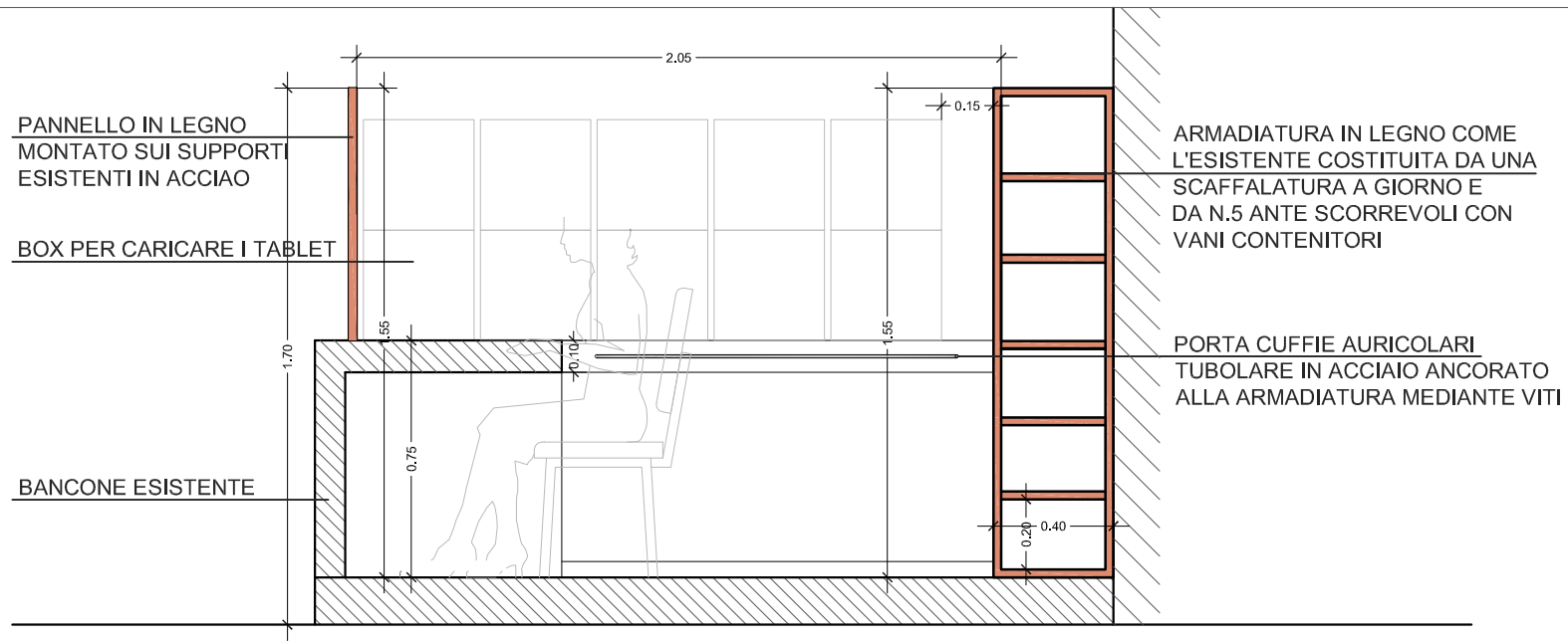
SEZIONE AA
