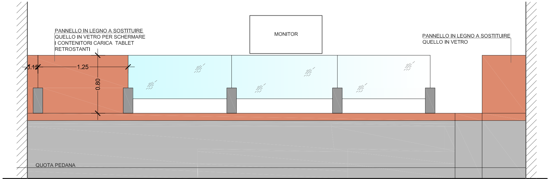
PROSPETTO
