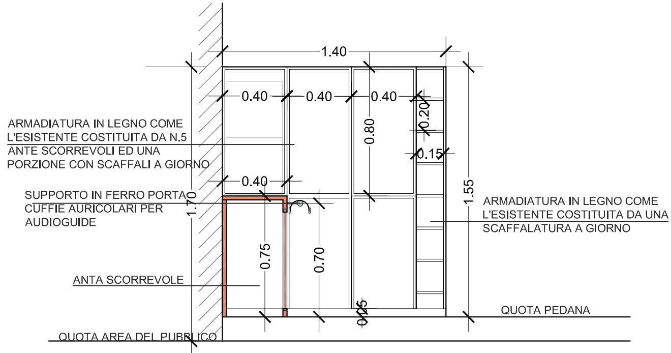
SEZIONE AA
