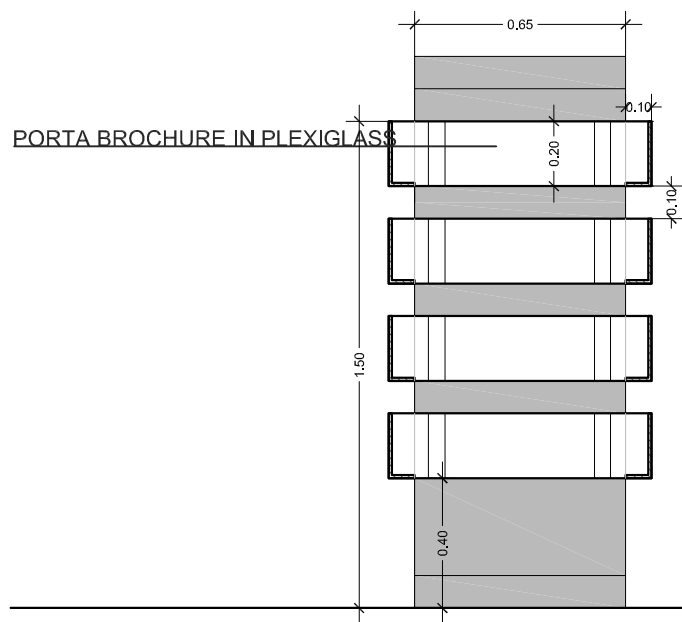
PROSPETTO 2
