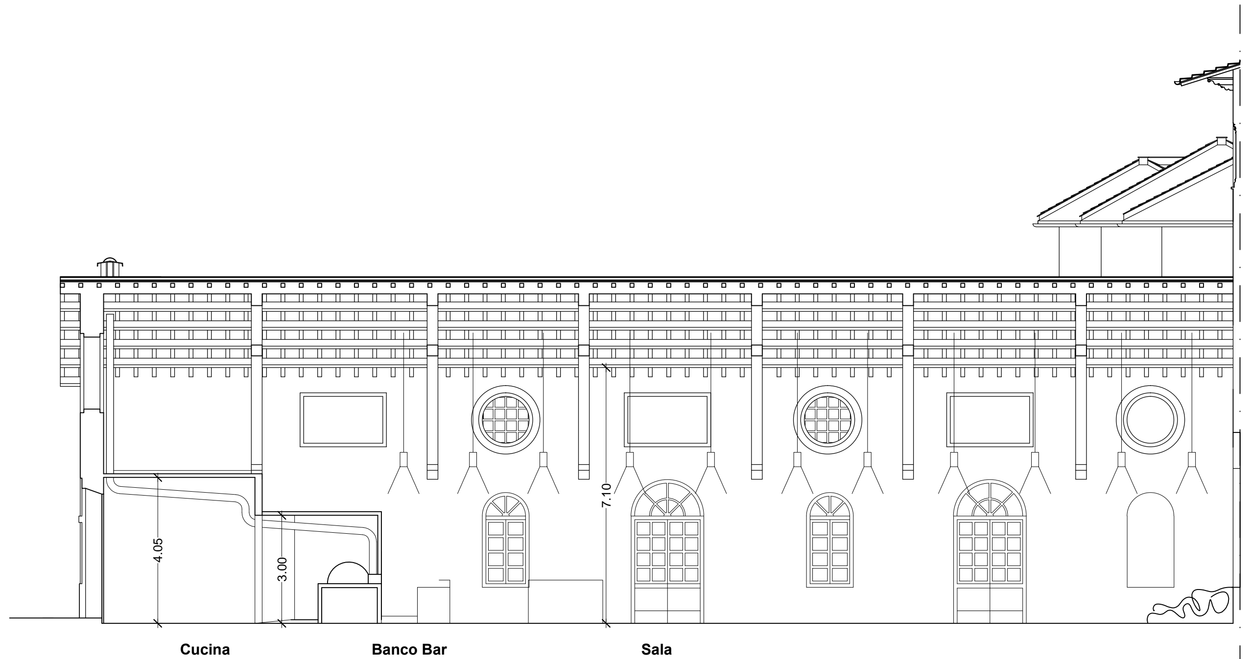
SEZIONE AA
